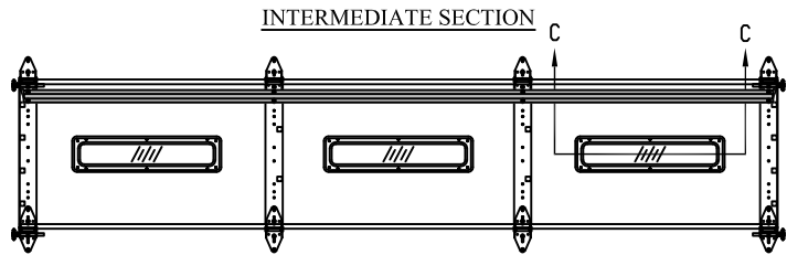
OPTIONAL GLAZED SECTION W/ 24" X 6" WINDOW LAYOUT N.T.S.
